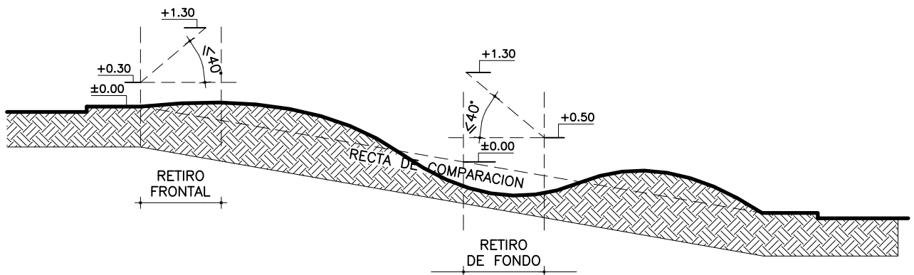
CORTE A-A
