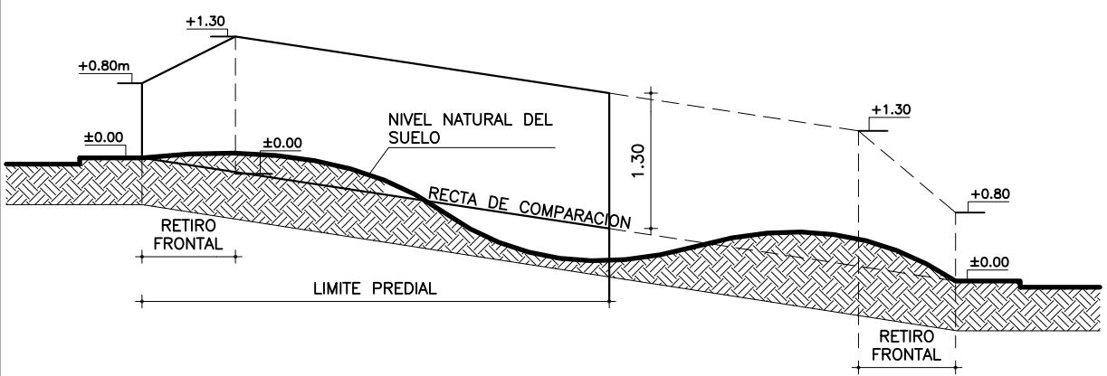
CORTE A-A
