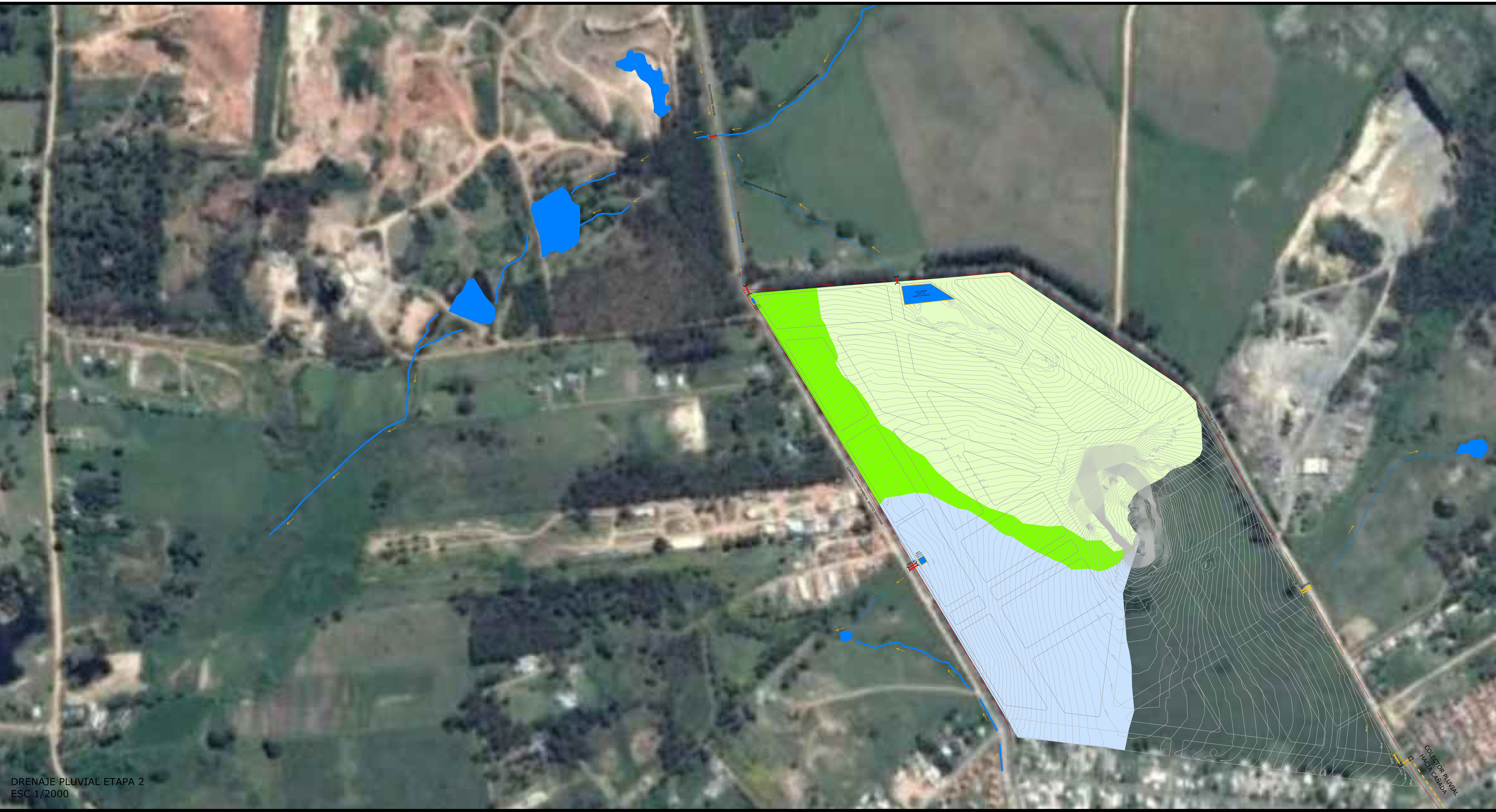
PLANTA DE UBICACIÓN S/ESCALA
